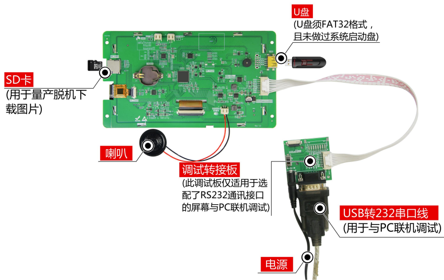
图 1-5 调试工具图
