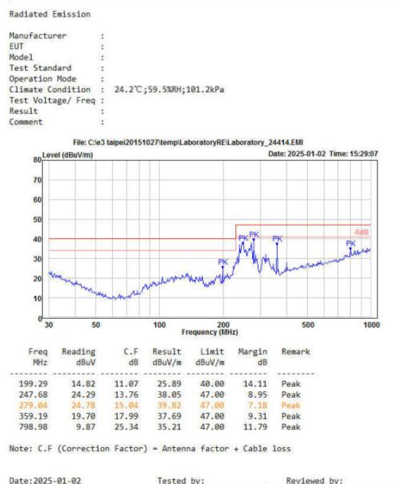
图 5-6 辐射测试水平方向
