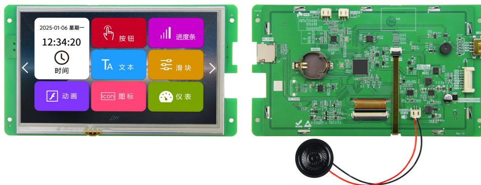
图 1-1 7.0 寸电阻触摸参考图
